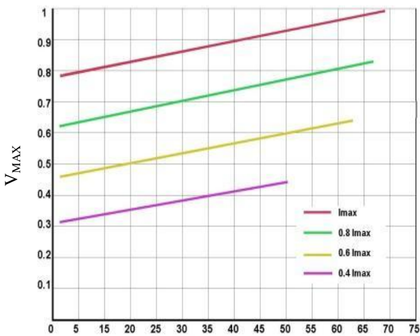
图4. V_{MAX} 与DT的关系图
