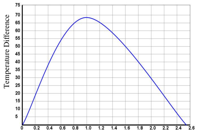
图3. DT与 I_{MAX} 的关系图
