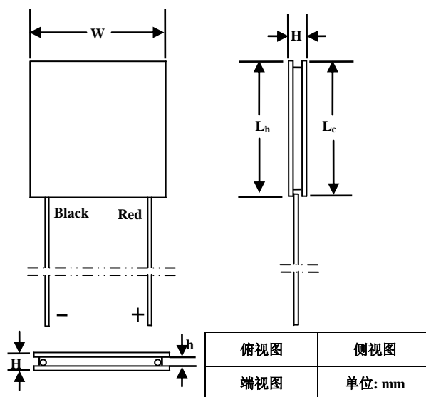
图6. 密封ATE1-161的机械尺寸图
