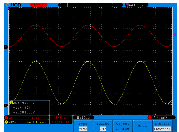
图 9、 f = 20kHz
