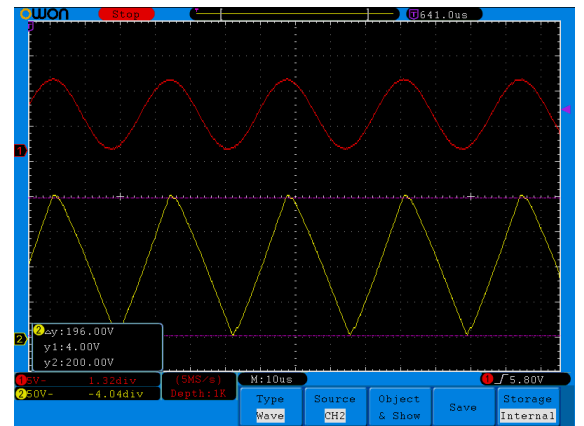
图 10、 f = 35kHz
