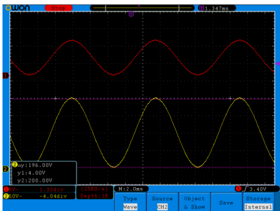
图 7、 f = 100Hz
