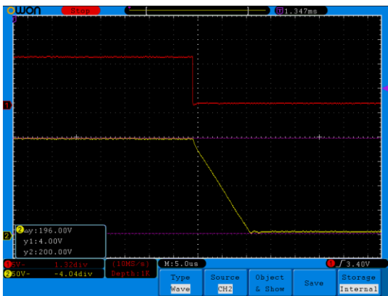
图 6、下降沿
