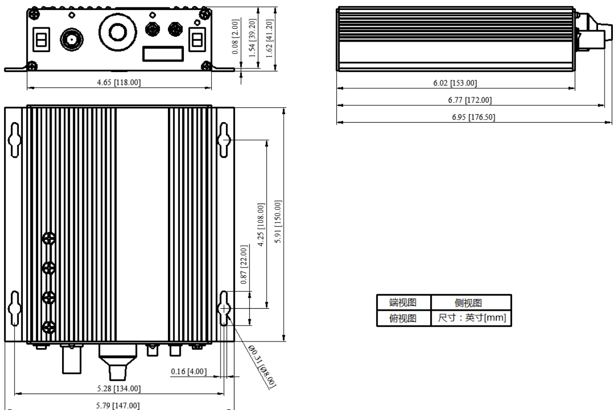
图12、AHVA2KV2X20MA的尺寸图
