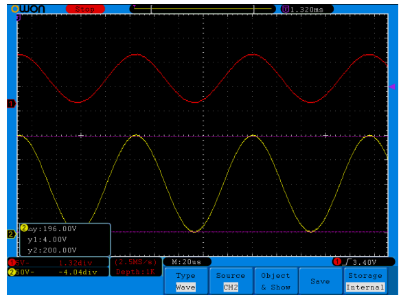
图 8、 f = 10kHz
