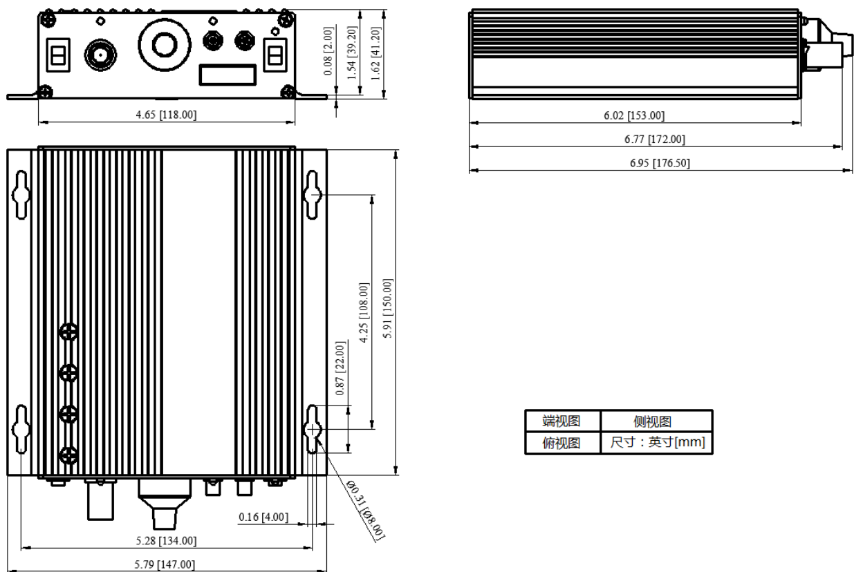
图12、AHVA2KV2X10MA的尺寸图
