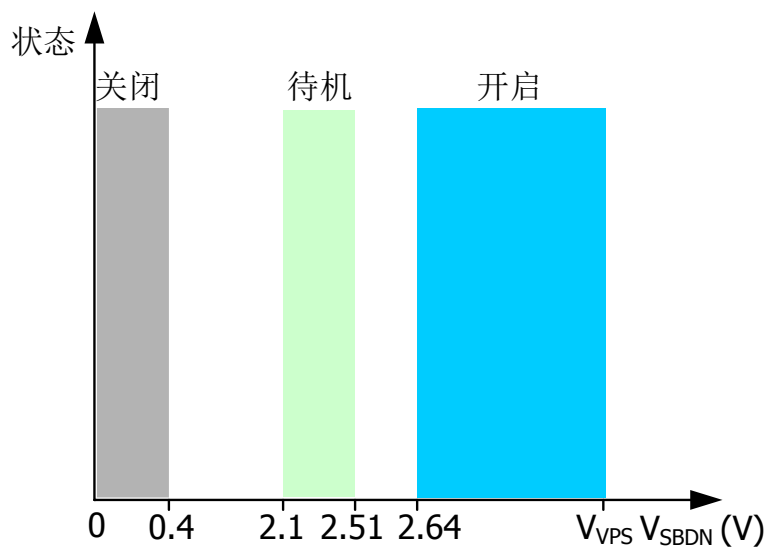
图 3、 V_{\text{SBDN}} VS. 放大器状态
