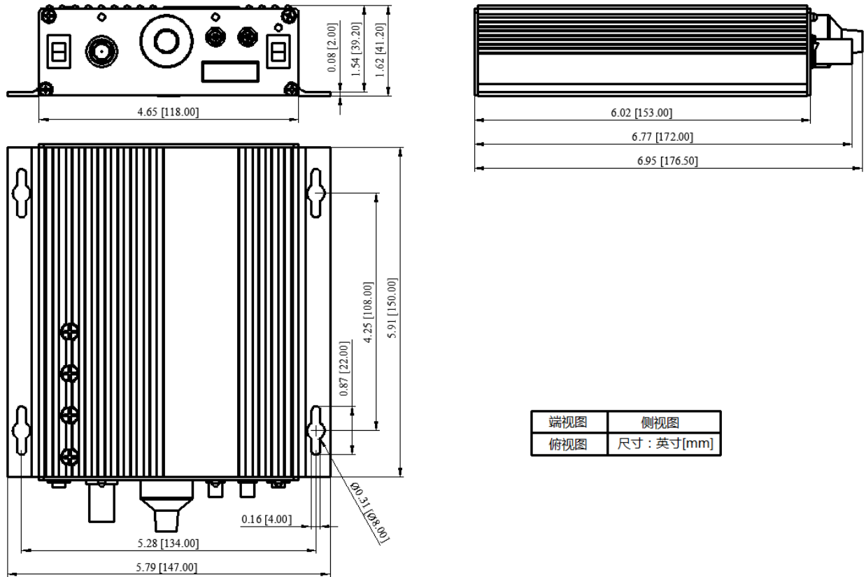
图5、AHVA100V2X50MA的尺寸图
